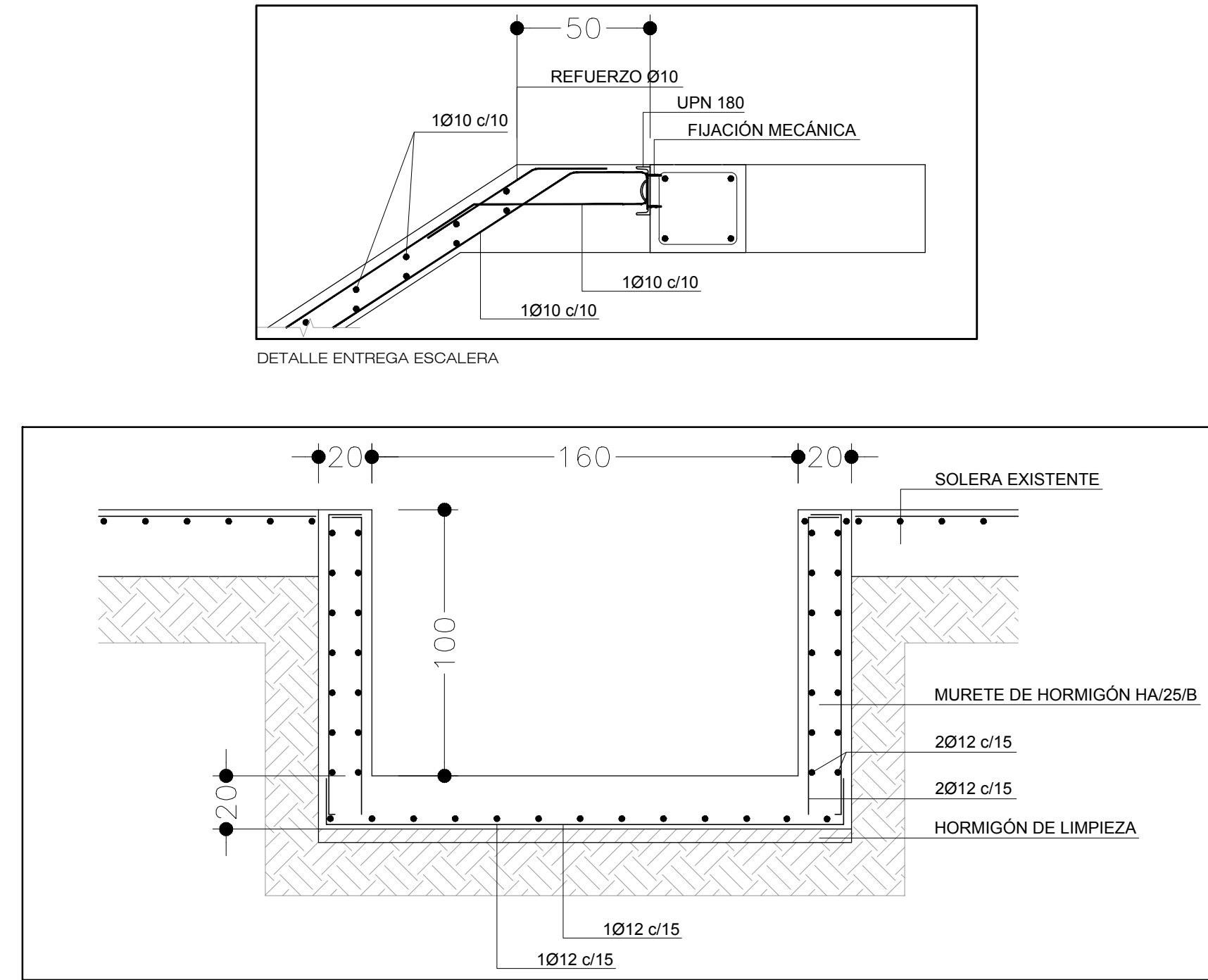
DETALLE FOSO ASCENSOR
