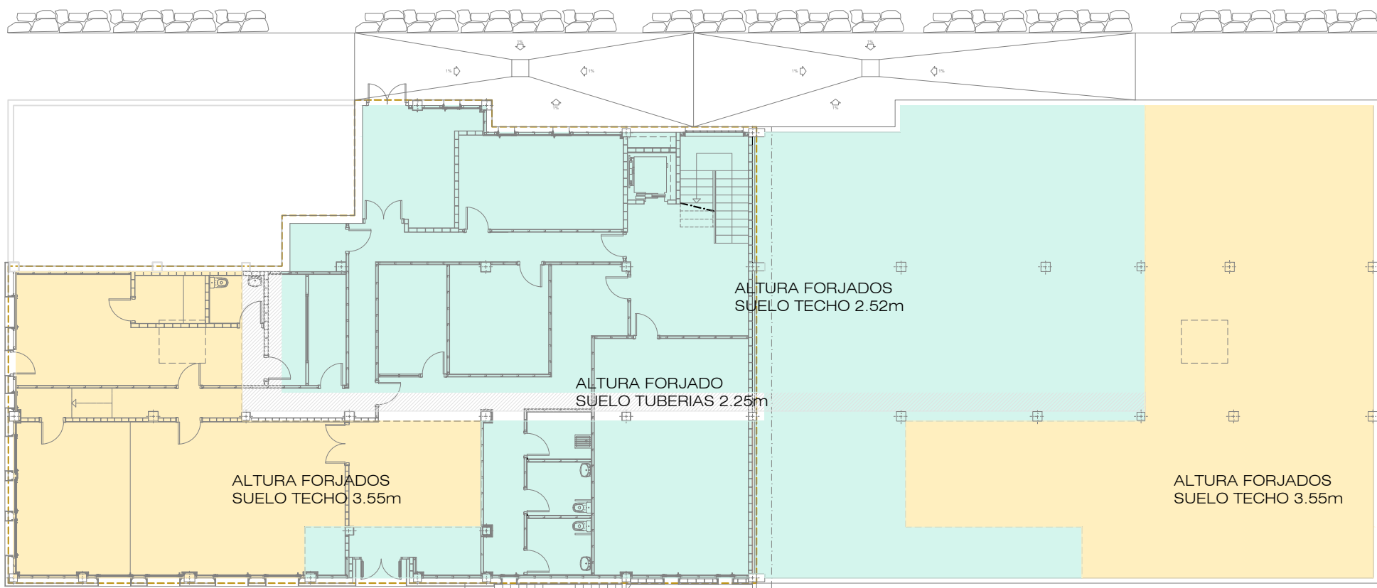
NIVEL INFERIOR (-2.87m)
