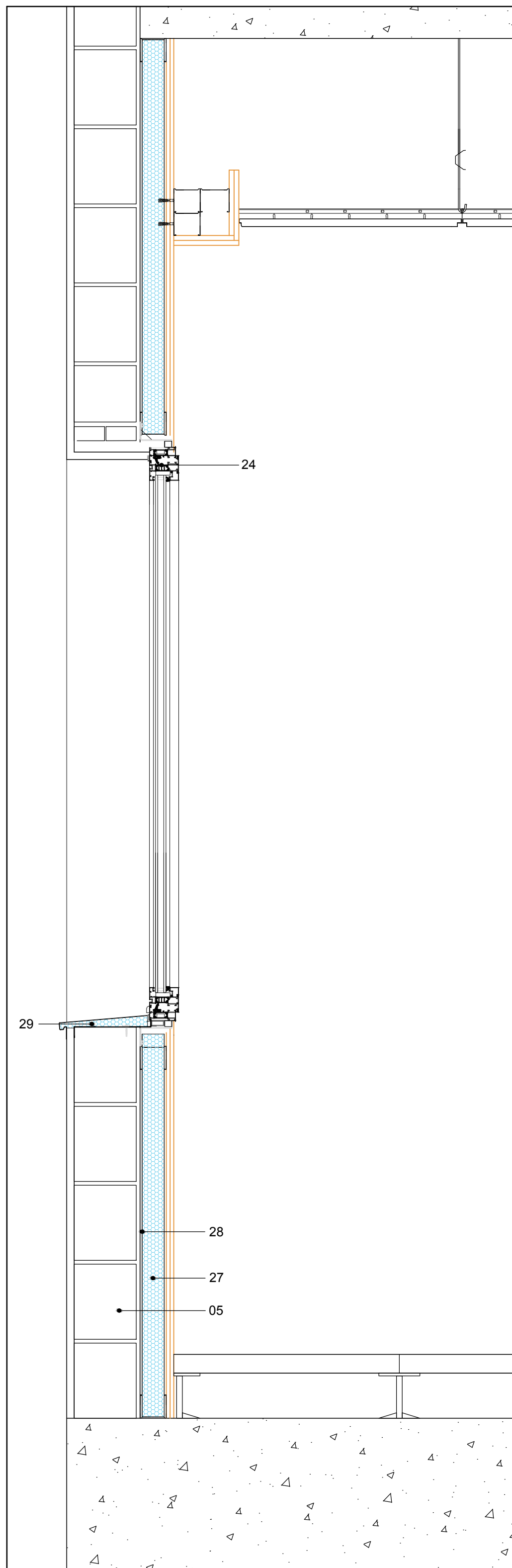
DETALLE 3
