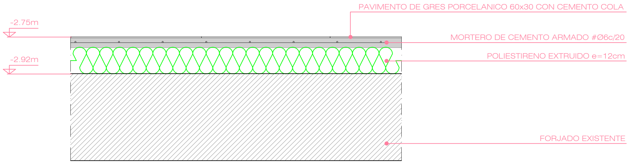
DETALLE DE RECRECIDO ALTURA 17cm
