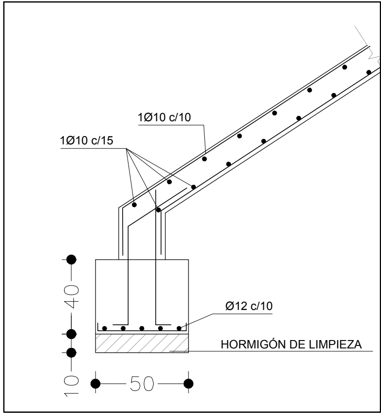
DETALLE ARRANQUE ESCALERA
