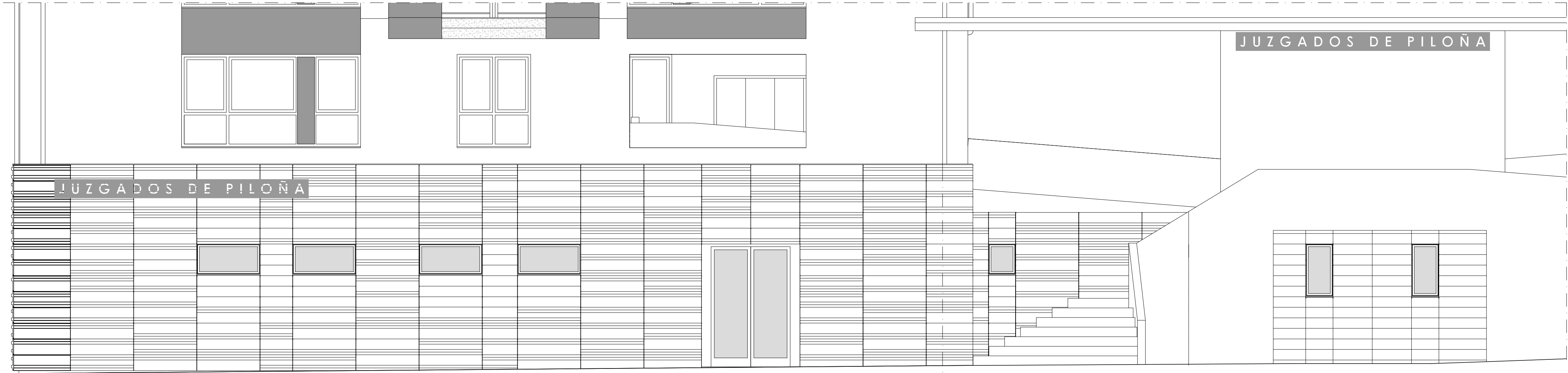
ALZADO ESTE NIVEL INFERIOR (-2.87m)
