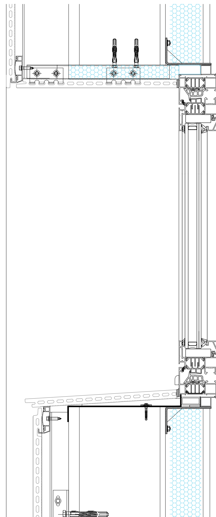
SECCION VENTANA, TIPO COR 70 CC16 RPT o SIMILAR ACRISTALAMIENTO SOLARLUX o SIMILAR 4+4/12/6 mm
