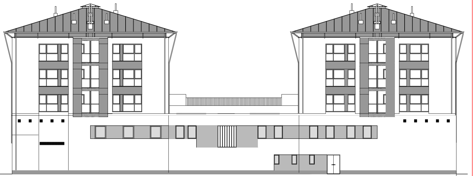
ALZADO OESTE NIVEL SUPERIOR (+0.17m) Y NIVEL INFERIOR (-2.87m)
