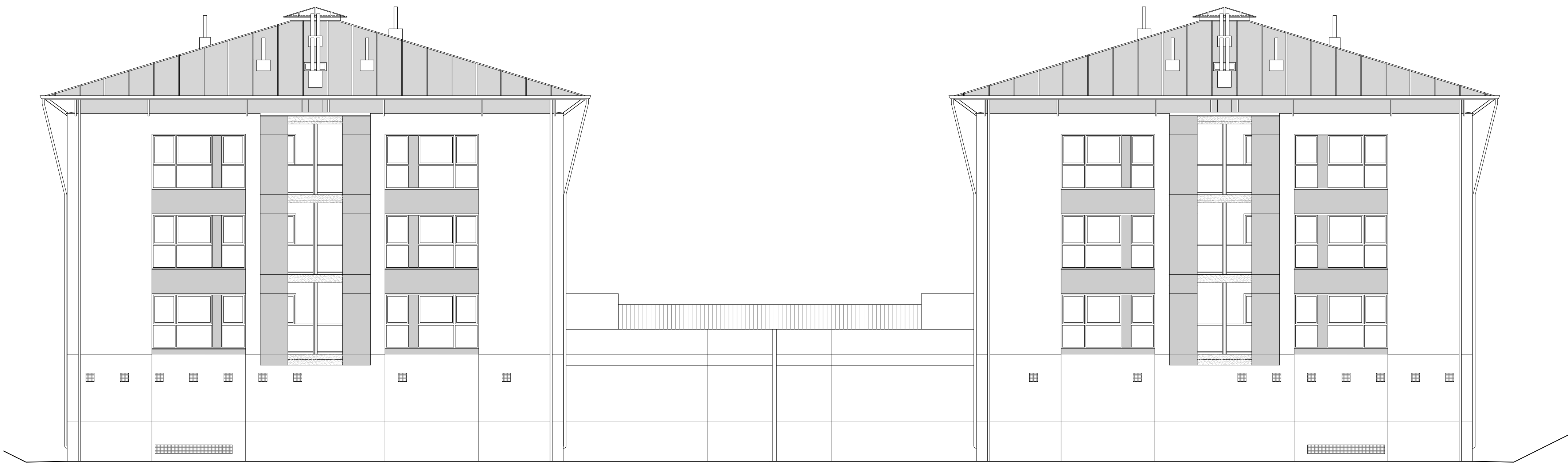
ALZADO OESTE
