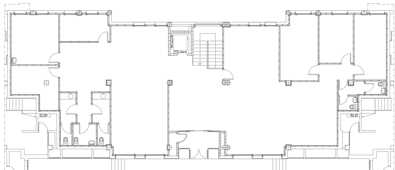
NIVEL SUPERIOR (0.17m)
