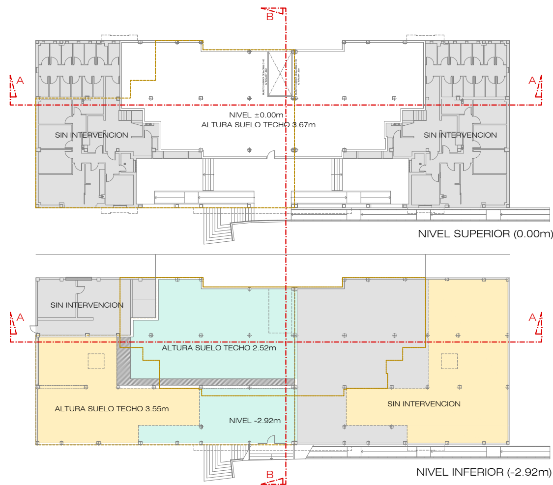
PLANTAS DE ORIENTACION
