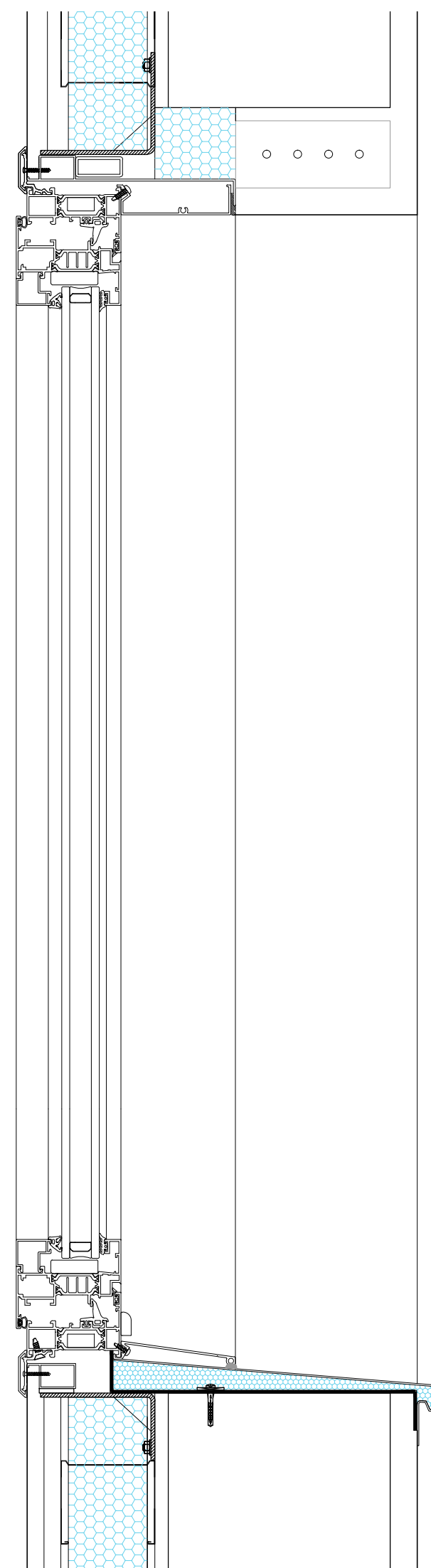
SECCION VENTANA, TIPO COR 70 INDUSTRIAL RPT o SIMILAR ACRISTALAMIENTO SOLARLUX o SIMILAR 4+4/12/6 mm
