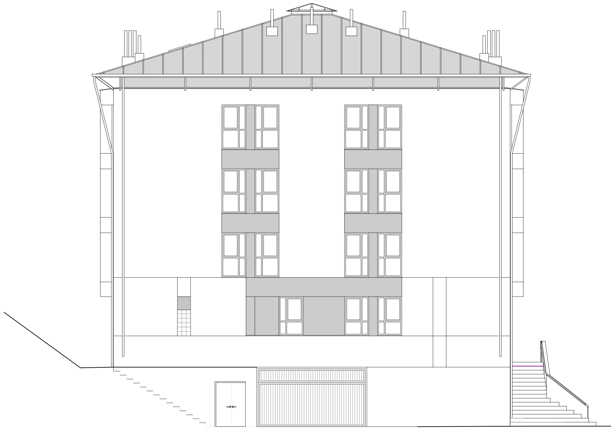
ALZADO SUR
