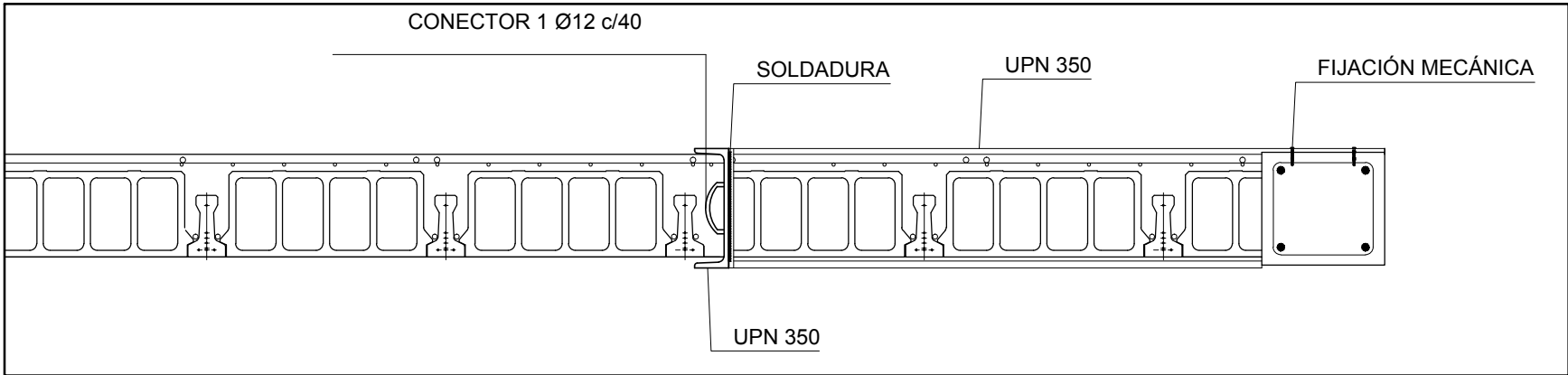
DETALLE 1-1
