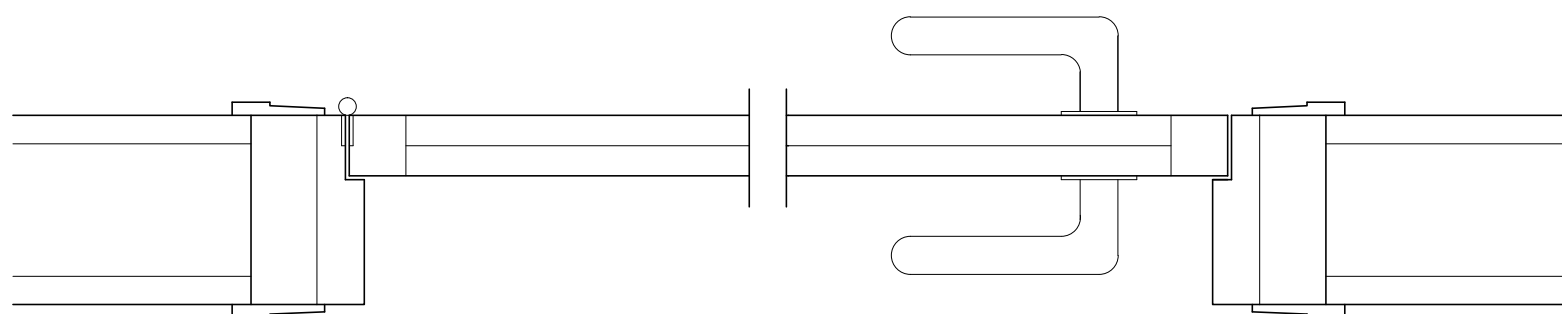
SECCION PUERTA DE TABLERO AGLOMERADO REV. RECHAPADO EN MADERA NOBLE ESCALA 1:4
