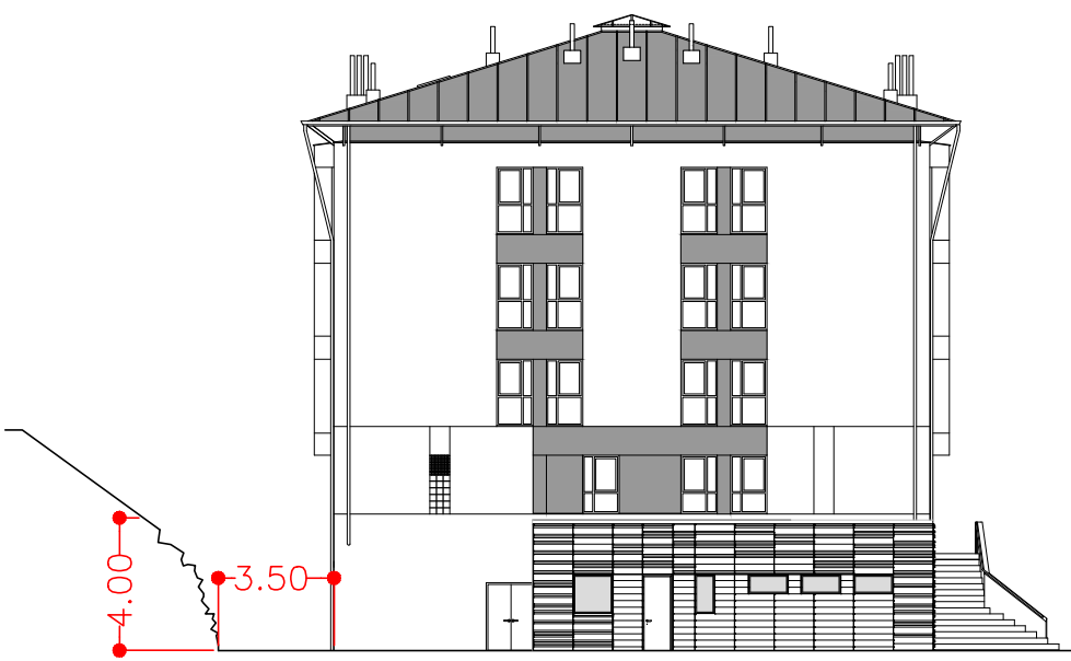
ALZADO SUR NIVEL SUPERIOR (+0.17m) ( Y NIVEL INFERIOR (-2.87m)
