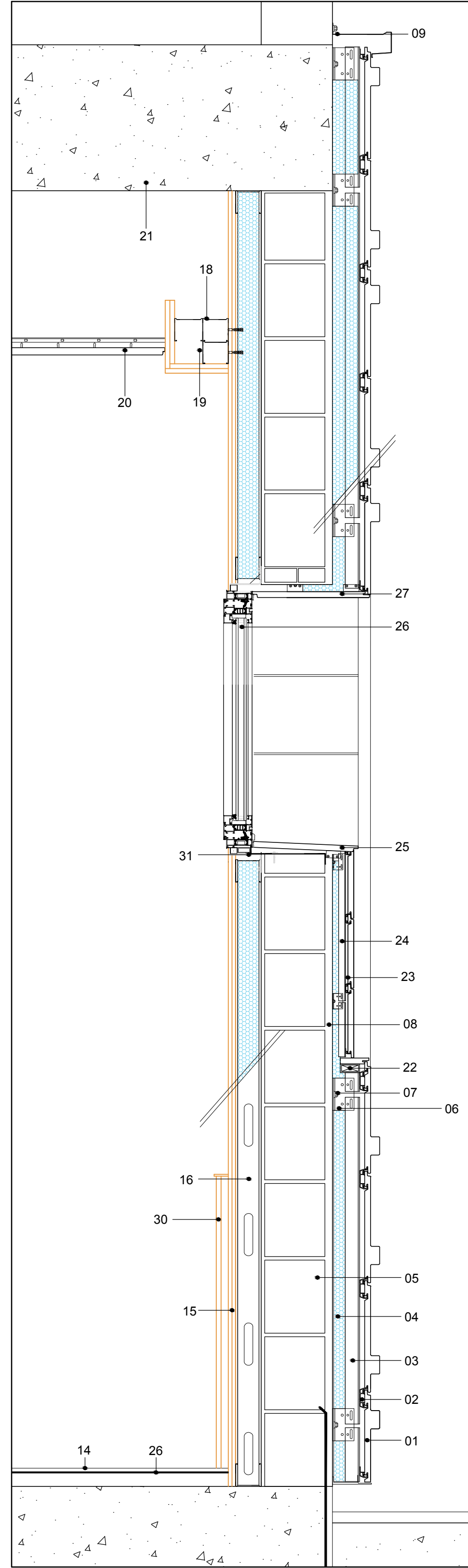
DETALLE 2
