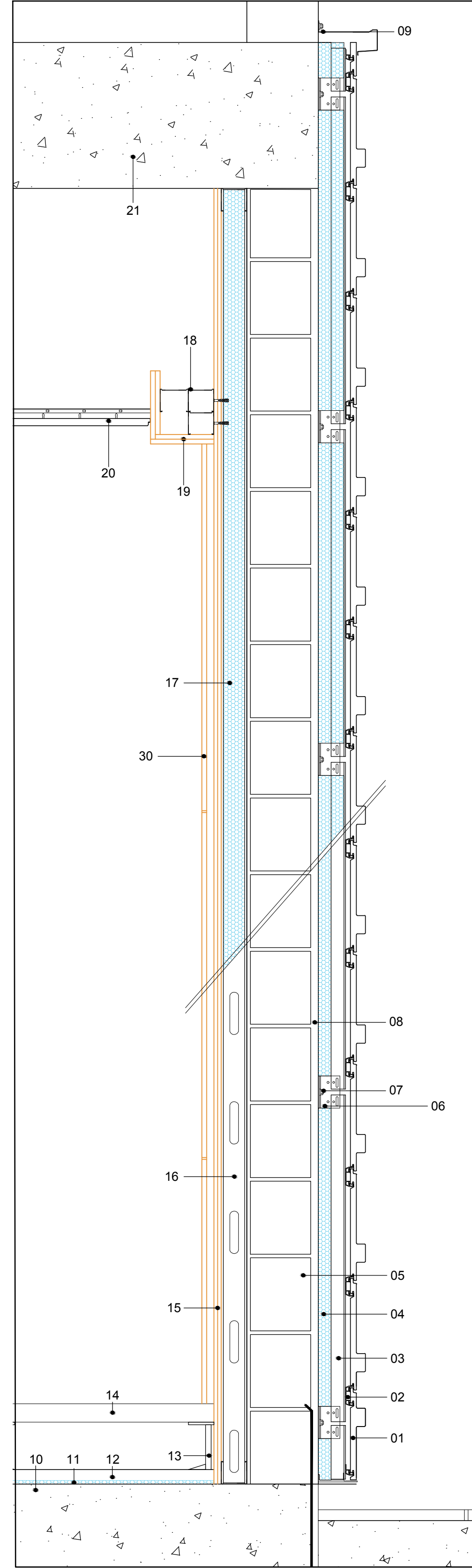
DETALLE 1
