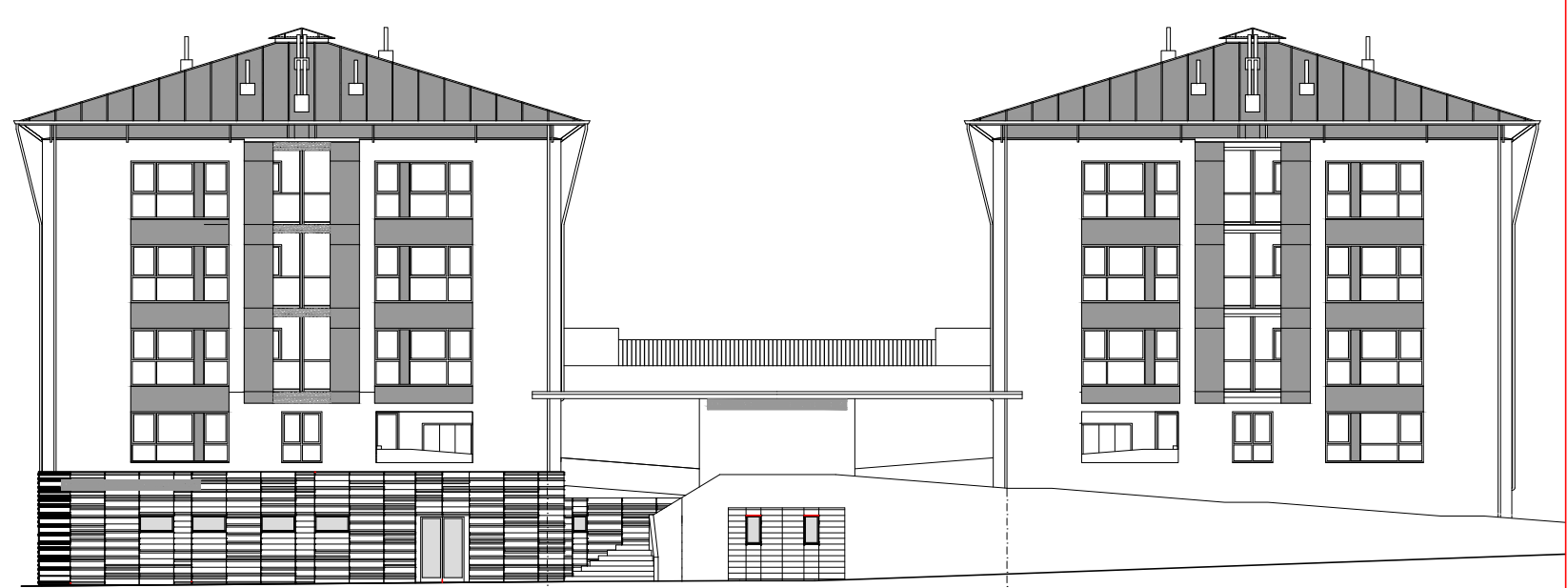
ALZADO ESTE NIVEL INFERIOR (-2.87m)
