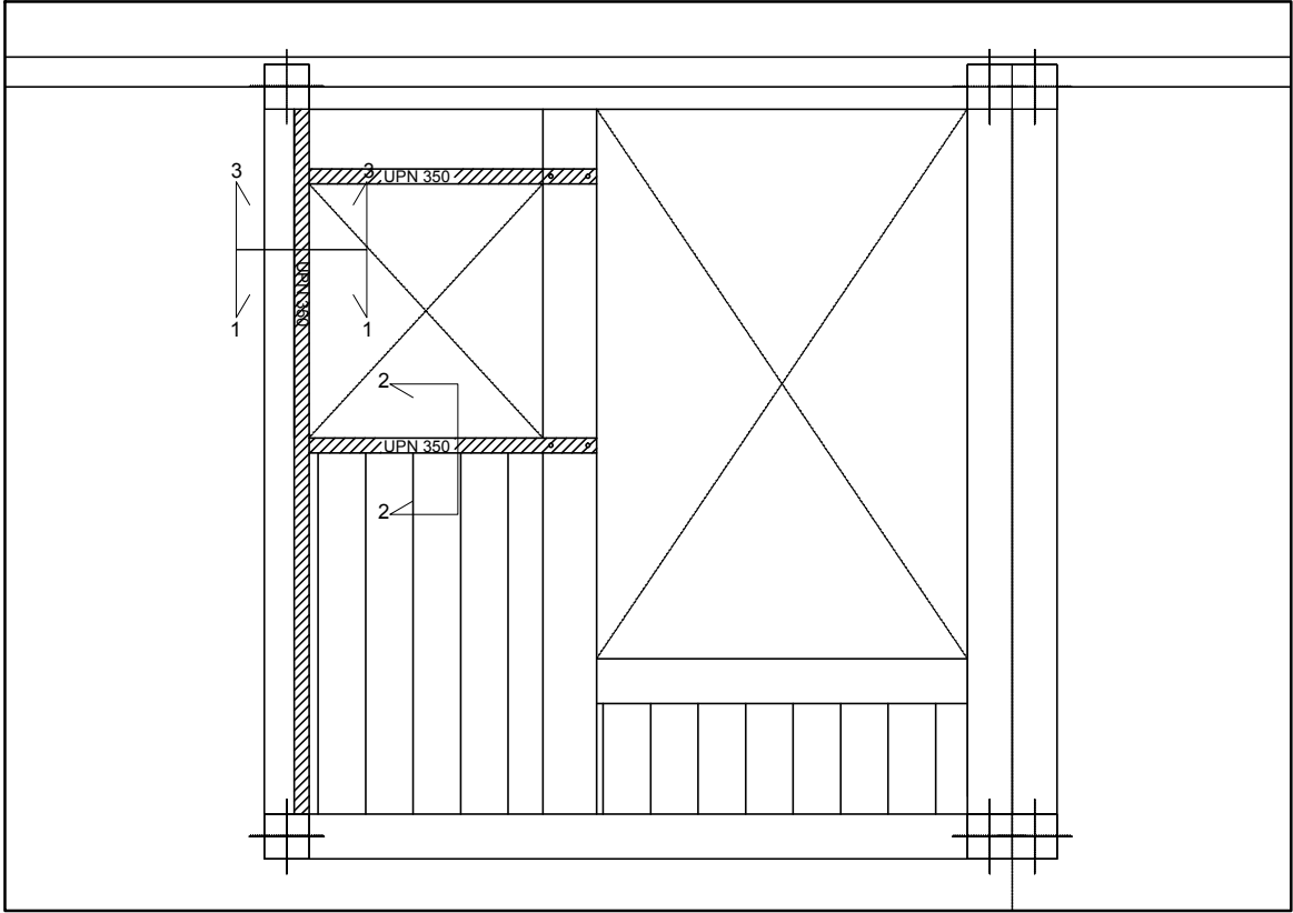
DETALLE ARRANQUE ESCALERA
