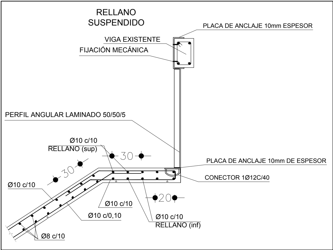
DETALLE DESCANSILLO
